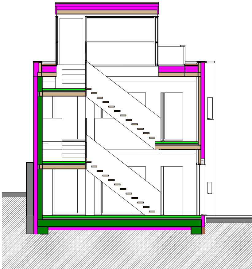
QUERSCHNITT
